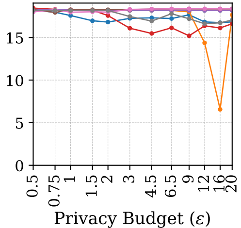
Brightkite
