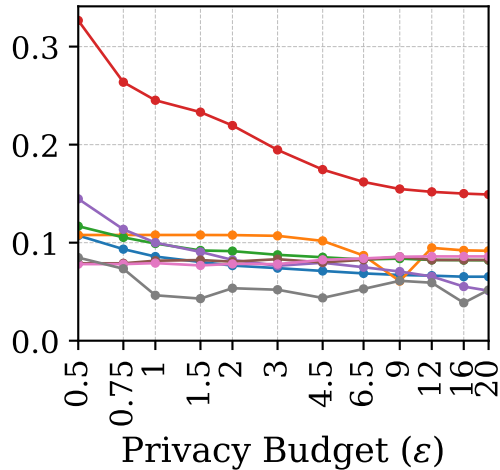
Facebook
